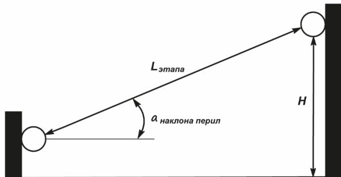
Схема: Подъем-спуск по наклонной переправе
