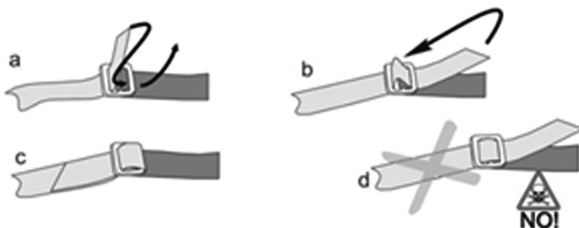
Рис. 2. Использование двухщелевых пряжек
