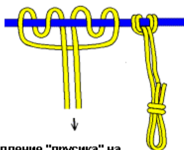
Крепление "прусика" на вертикальных перилах
